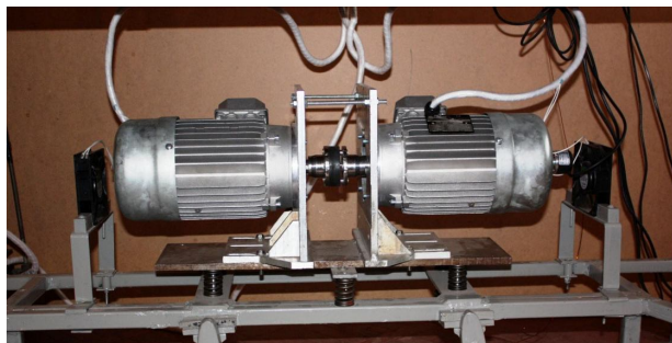
Рисунок 2 – Лабораторний електромеханічний комплекс
