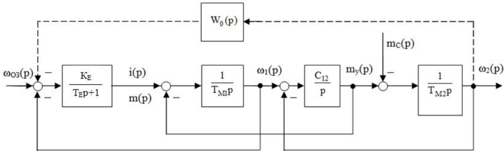
Рисунок 2 – Структурная схема электропривода при электромеханическом взаимодействии подсистем
