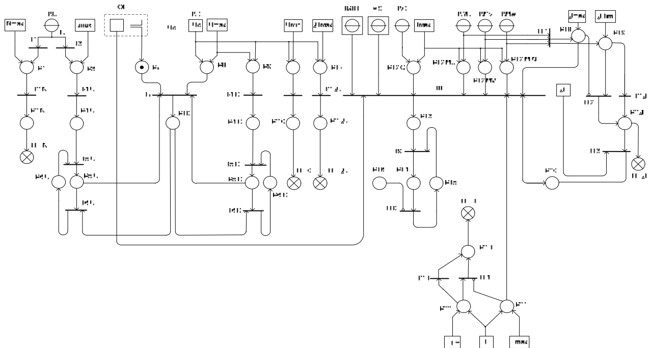
Рисунок 4 – Обобщенная сеть Петри системы защиты от аномальных ситуаций тягового электропривода переменного тока рудничного контактного электровоза
