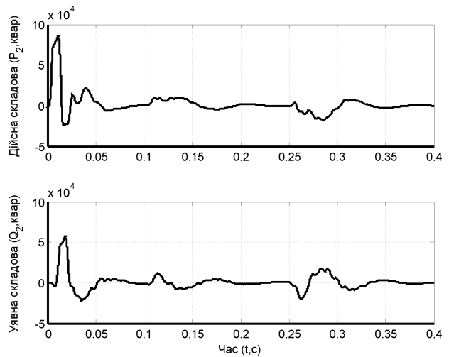
Рисунок 5 – Графіки перехідних процесів складових умовної потужності зворотної послідовності під час симетрування навантаження з використанням ПІ-регуляторів
