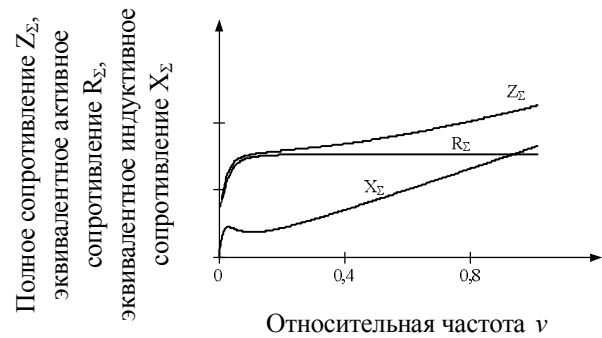
Рисунок 2 – Графики зависимостей от относительной частоты полного, активного и индуктивного сопротивлений Т-образной схемы замещения
