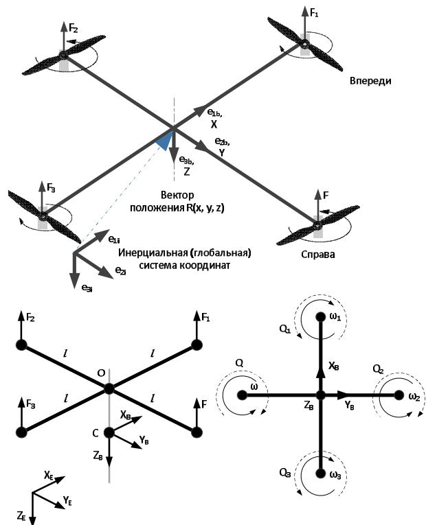
Рисунок 1 – Схема усилий и системы координат квадрокоптера
